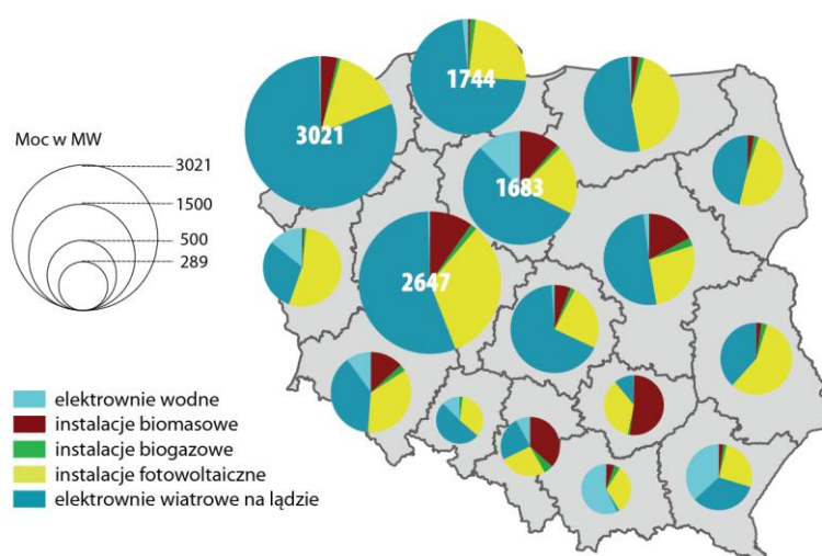
Rysunek 22. Moc elektryczna instalacji OZE powyżej 50 kW według województw z podziałem na technologie w MW, stan na 31 grudnia 2023 r.
